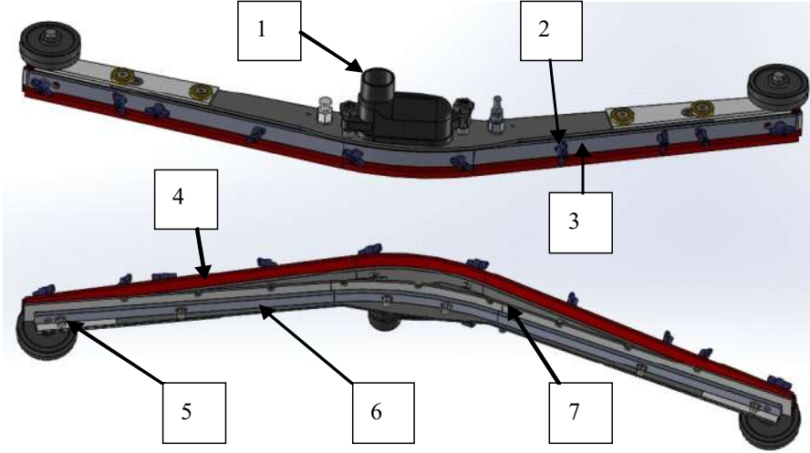
Şekil 31 (SIYIRICI MEKANİZMA)
